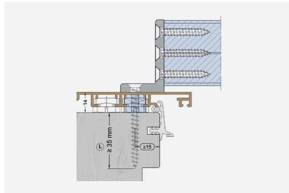
FPA HOLZ-ALUMINIUM 18 MM
