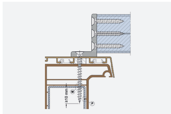
FPA KUNSTSTOFF-ALUMINIUM-FENSTERSYSTEM
